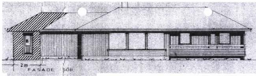
Påbygg Fasade sør -Påbygg er skravert -Dør merket B ny dør, størrelse 80/210
