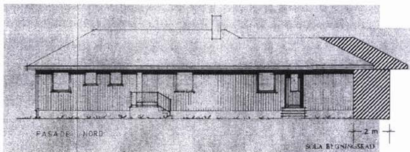
Påbygg Fasade nord -Påbygg er skravert
