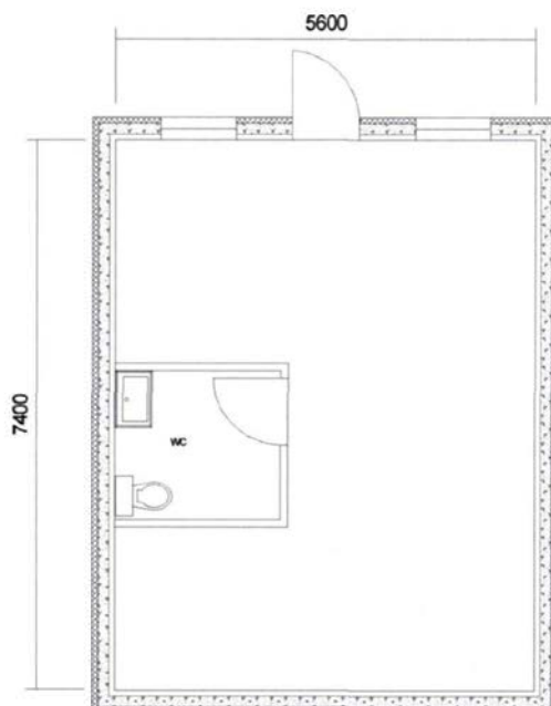
Kjeller/Hobbyrom BRA 41,4
