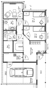
U. etasje
