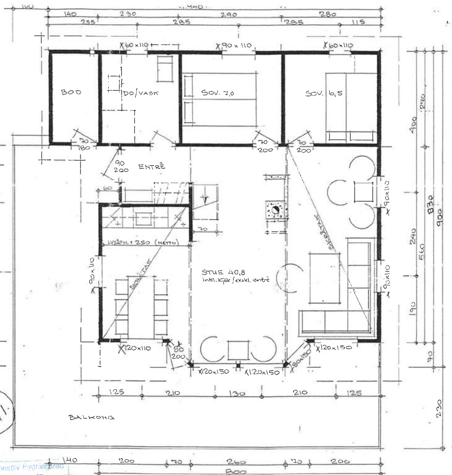
HOVEDETASJEPLAN - Brutto Gr.f. = 71,53 m 2 + BALKONG - M = 1:50
