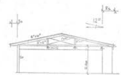
SKITZ A-A.
