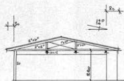
SNITT A-A.
