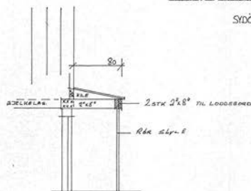
DETALJ B-B.
