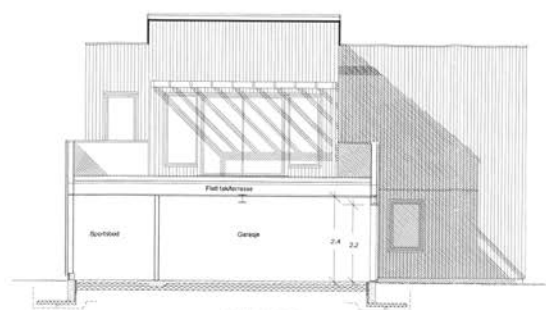
SNITT B-B
