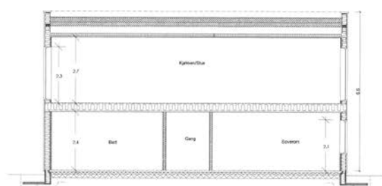
SNITT A-A
