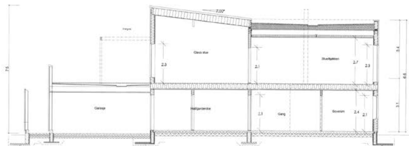
SNITT C-C
