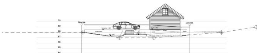
FASADE MOT NORD TERRENGPROFIL 5
