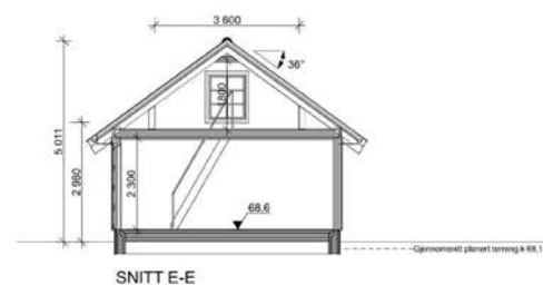
SNITT E-E
