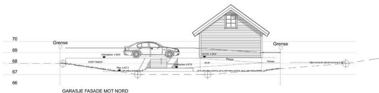
GARASJE FASADE MOT NORD
