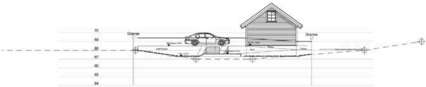
FASADE MOT NORD TERRENGPROFIL 5
