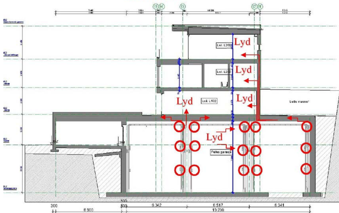
Figur 12: Prinsipp for flanketransmisjon (overføring av strukturlydlyd) i parkeringsanlegg BK2 (Hus L), snitt C. Dette er et utsnitt fra figur 3 (Tegning I_a29_02_snitt_og_fasader_pdf, lastet ned fra Asker kommune)
