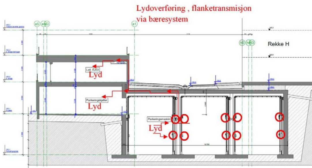
Figur 11: Prinsipp for flanketransmisjon (overføring av strukturlyd), parkeringsanlegg BK1 (Hus E). Dette er et utsnitt fra figur 1 (e_a29_02_snitt_og_fasader_pdf, lastet ned fra Asker kommune).
