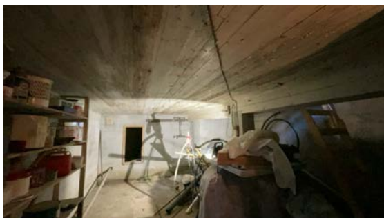
Utført fuktmålinger på himlingsbord mot bjelkelag. Påvist forhøyet fuktprosent.
