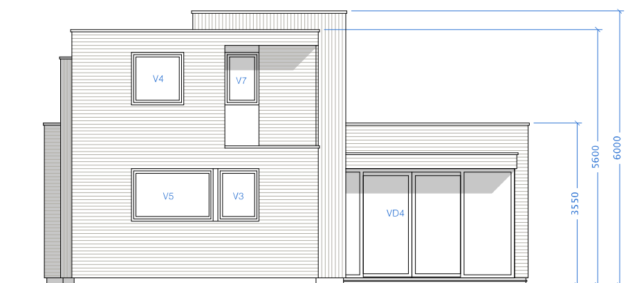
fasade nord - standard
