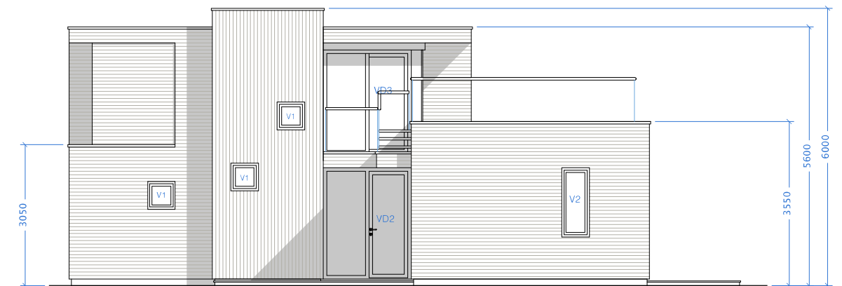
fasade vest - m/ takterasse
