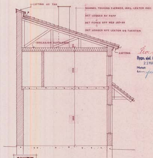
SNITT
