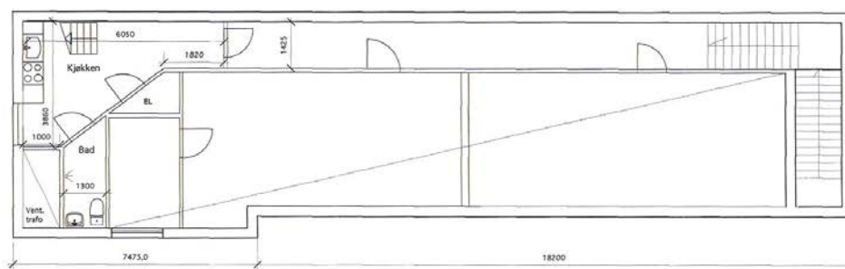
PLAN 2. ETG.
