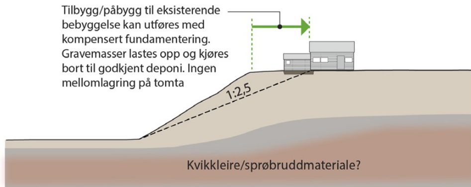
Figur 6 Grønn pil angir hvor tilbygg/påbygg kan bygges uten geoteknisk vurdering, forutsatt kompensert fundamentering
