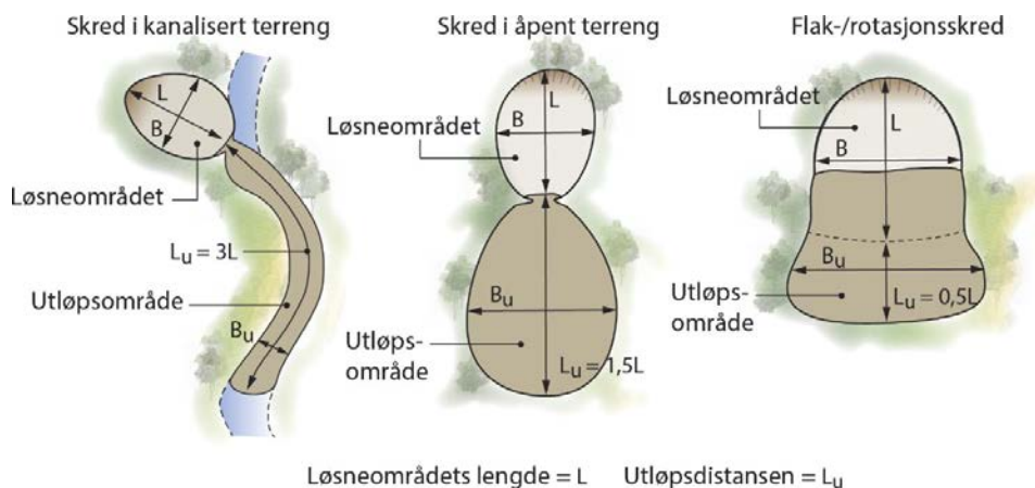
Figur 4.10. Sammenheng mellom løsningsområdets lengde, L , og utløpsdistansen, L_u (34)
