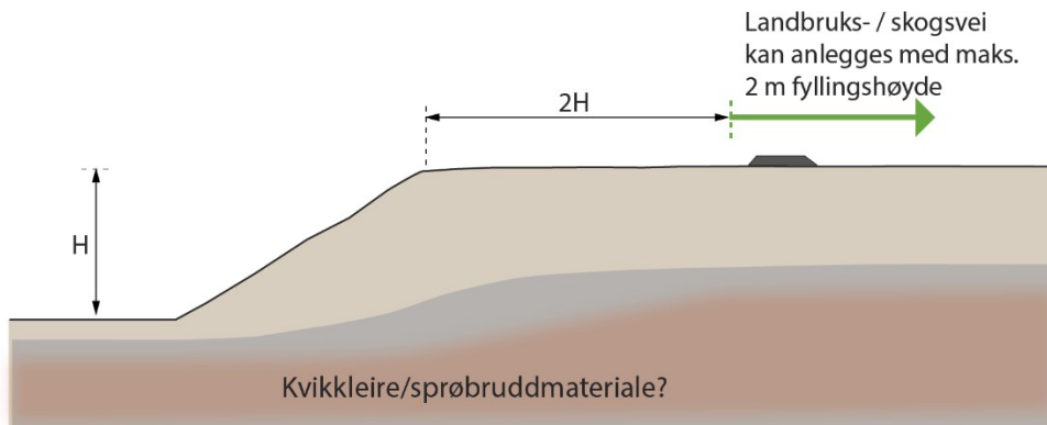
Figur 12 Landbruks-/skogsvei kan plasseres på toppen av skrånning bak 2H forutsatt ingen fyllingshøyde < 2 meter
