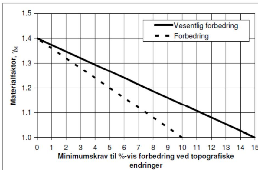
Figur 4.1 Krav til prosentvis forbedring ved topografiske endringer [2]
