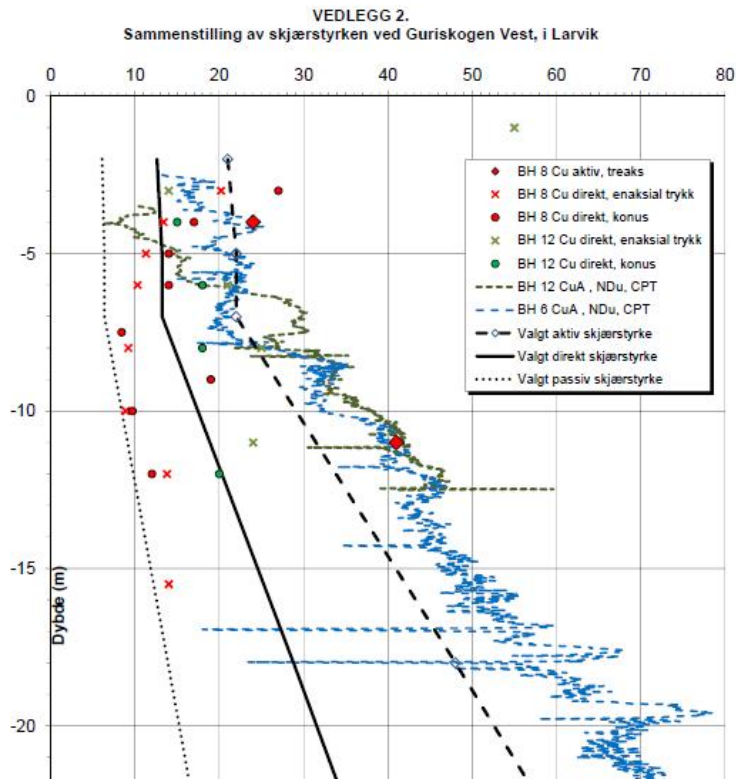
Figur 4.2 Valgt C_u -profil, basert på sammenstilling av utførte undersøkelser.
