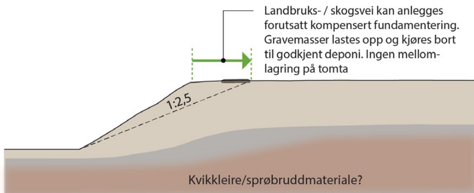
Figur 14 Landbruks-/skogsvei kan plasseres på toppen av skrånning innenfor 1:2,5-linja forutsatt kompensert fundamentering
