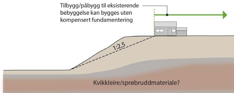
Figur 5 Grønn pil angir hvor tilbygg/påbygg kan bygges uten kompensert fundamentering eller geoteknikk vurdering
