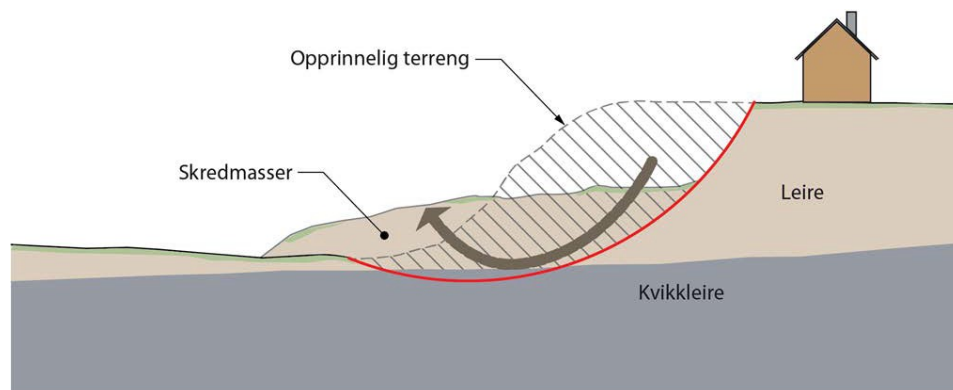
Figur 2.10 Prinsippkisse som viser rotasjonsskred.
