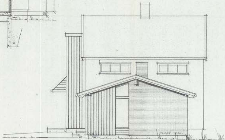
FASADE MOT ÖST
