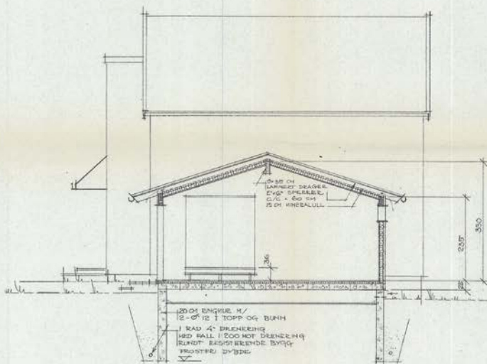
SNITT GJ. TILBYGG
