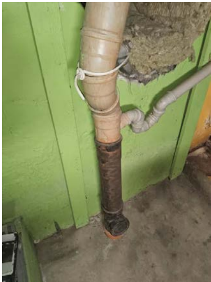
Avløpsrør med stakeluke i kjeller.
