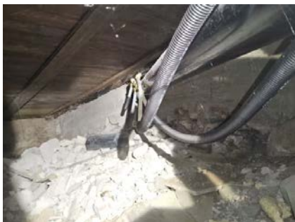
Åpen rørfordeling/koblinger i krypkjeller.
