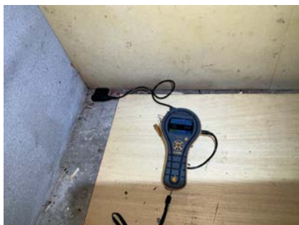
Fuktmåling med pigg i påforet vegg på mur i kjellerbod mot sør-øs. Fuktmåling viser 17,6% fuktinnhold i trevirke.
