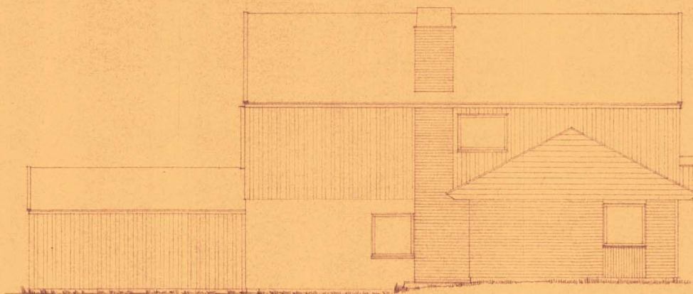
FREDRIKSHALDS KREDITBANK, BANKFILIAL. Fasade mot nord-øst. KNUT HEIN, ARKITEKT KHAL, SARPSBORG 3. NOV-61.
