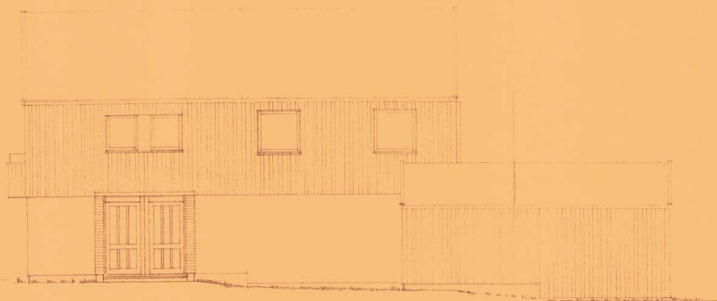
FREDRIKSHALDS KREDITBANK, BANKFILIAL. Fasade mod sydvest. KNUT WEIN, ARKITEKT MÅL, SÆRPSBORG, 3 NOV-61
