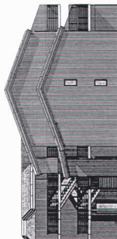
FASADE MOT NORDVEST
