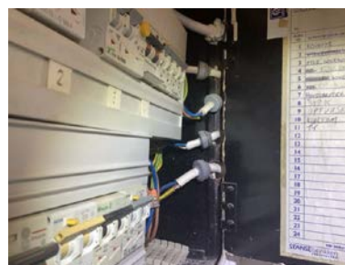
Utette kabelføringer i sikringsskap.
