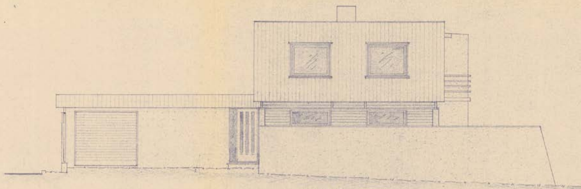
FASADE VEST
