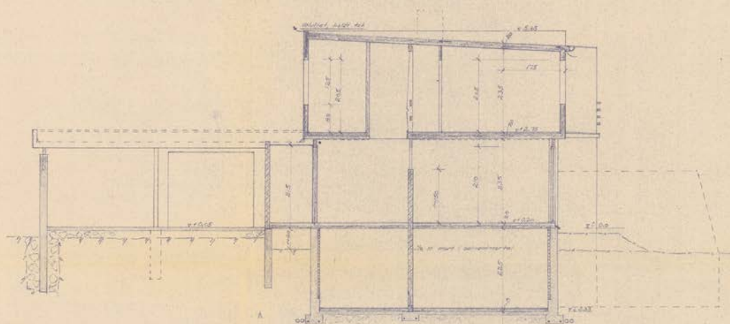
SNITT 1-1
