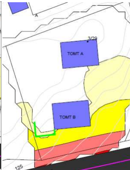
Figur 5: Beregnet L_{den} støynivå 1,5 m over terreng med støyskjermingstiltak.
