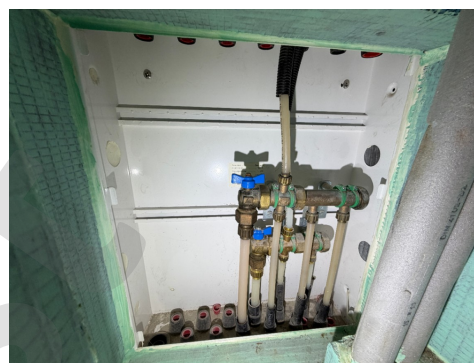
Rørskap i baderomsvegg med 2 x stoppekraner
