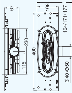
Slukdel sideutløp lav 40 og 50 mm.
