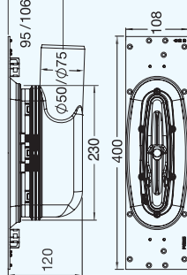
Slukdel gavelutløp Utløp Ø 50 og 75 mm.
