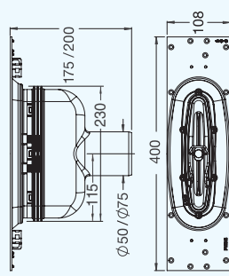
Slukdel bunnutløp Utløp Ø 50 og 75 mm.
