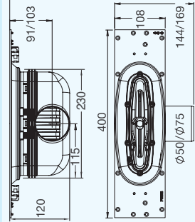
Slukdel sideutløp Utløp Ø 50 og 75 mm.
