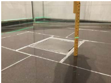
Målt fall til sluk. 20mm.
