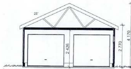
Snitt A-A
