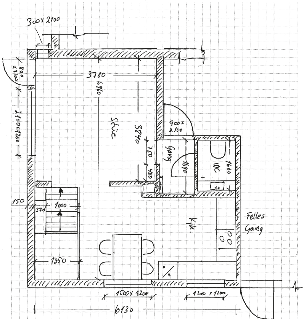
Snorresgt. 26 Plan 1. etasje
