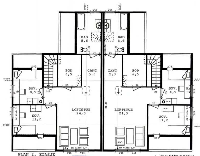
PLAN 2. ETASJE
