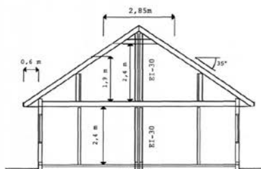
HOVEDSNITT B-B
