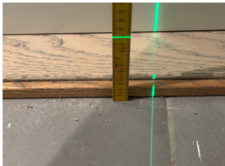
Fallforhold ca. 100 mm overkant gulv ved terskel
