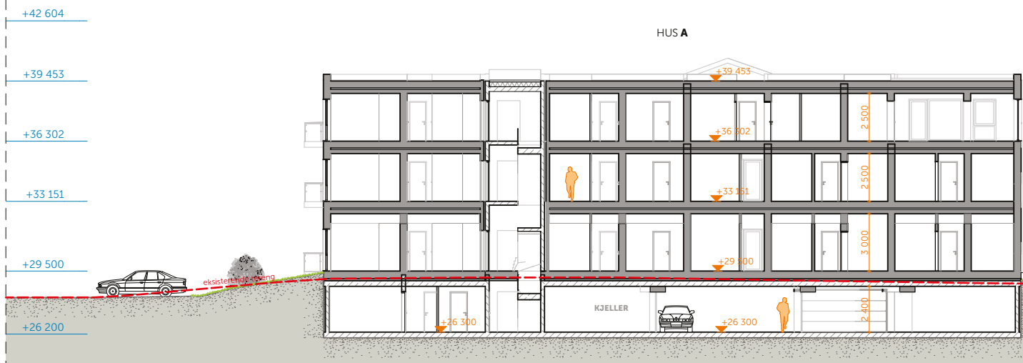
SNITT A-A 1:200
