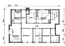
plan av underetasje.
