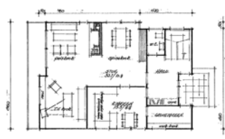
plan av tetasje.
