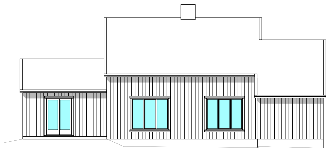
FASADE ØST
