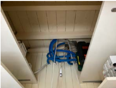
Samlestokk for rør i rør opplegg i bod i entre.
