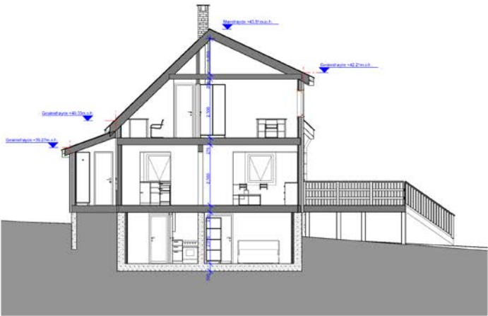
Snitt 1-1 1:100
