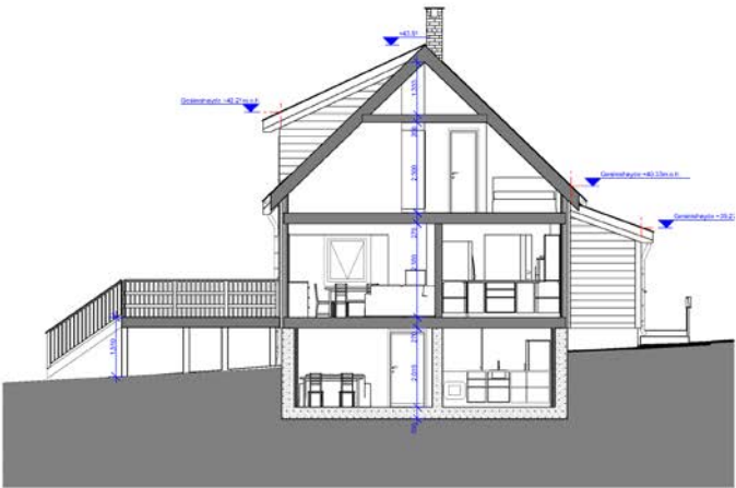
Snitt 2-2 1:100
