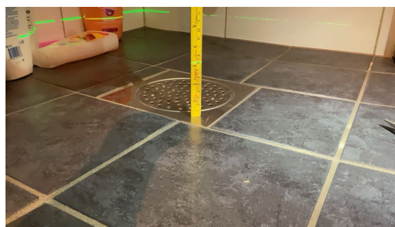
Målt fall til sluk: 31mm
