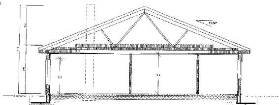
SNITT A-A
