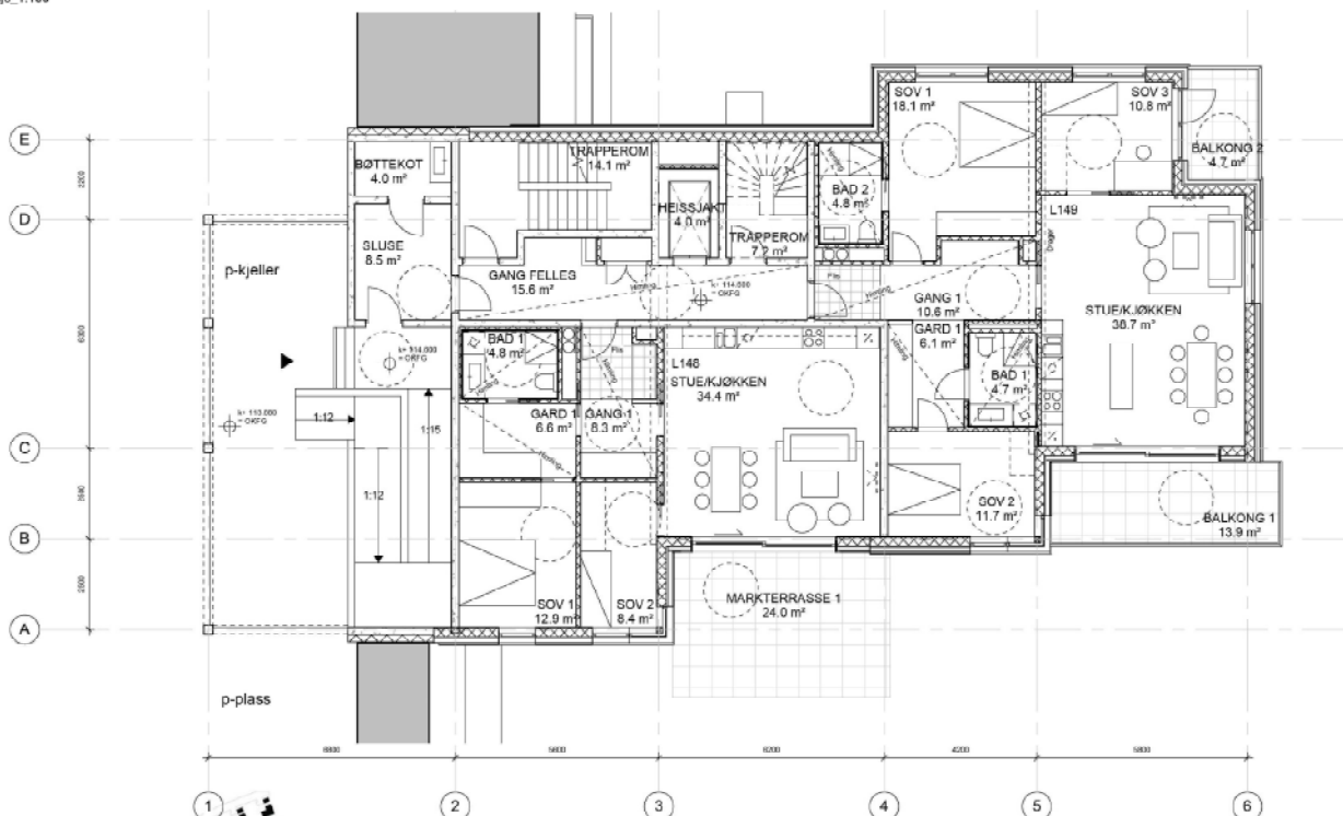
plan U1 etasje_1:100
