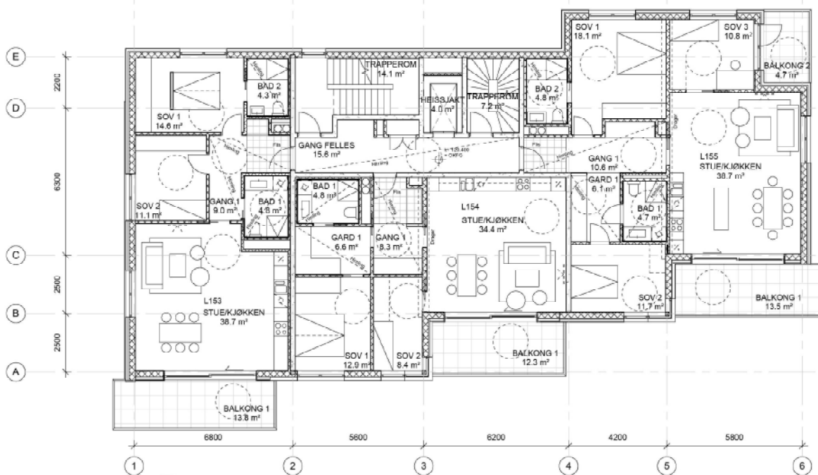
plan 02 etasje_1:100
