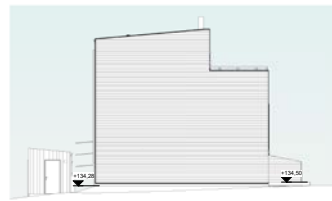
Rekke 9 - Fasade Vest
