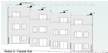
Rekke 9 - Fasade Syd
