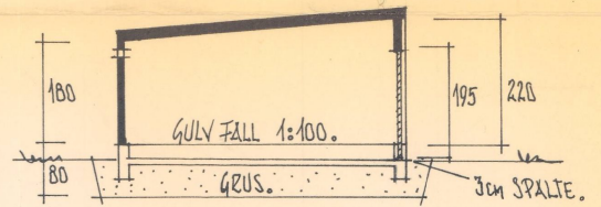
SNITT.
