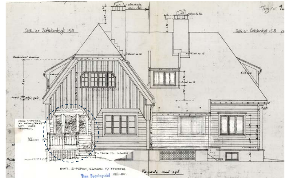
Figur: Påtegningen til venstre på fasadetegningen viser godkjent utforming av ny vinduer og veranda.
