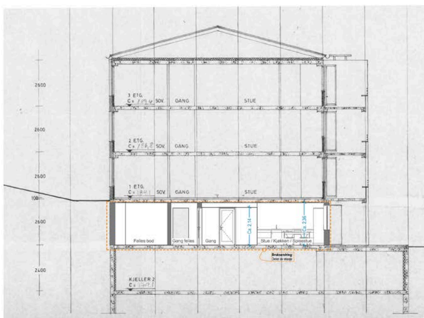
Lindebergåsen 49 / Snitt 01
