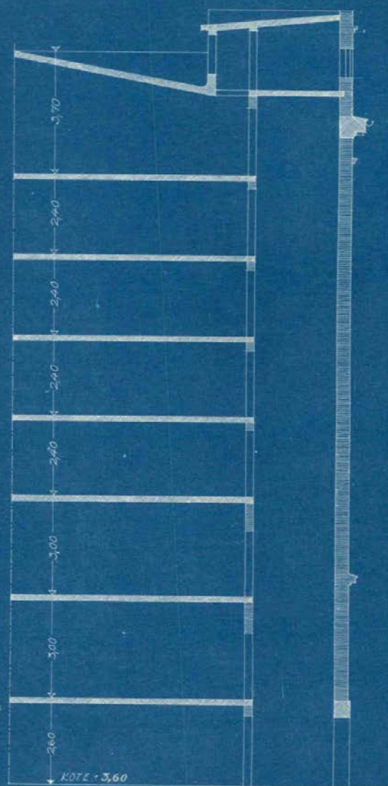
LÆNGDESNIIT
