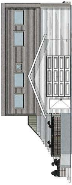
Fasade nord 1:100
