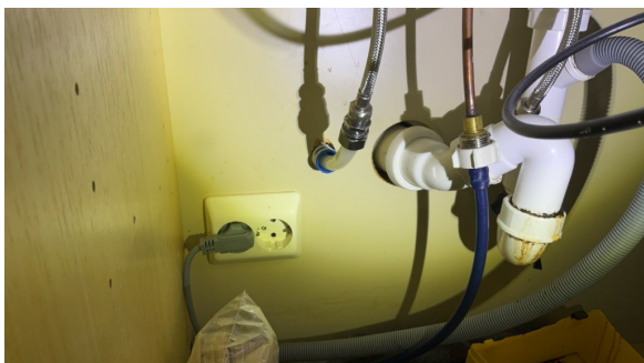
I kjøkkenskap er det ikke tett tilslutning mellom varerør og vannrør på rør i rør opplegget.
