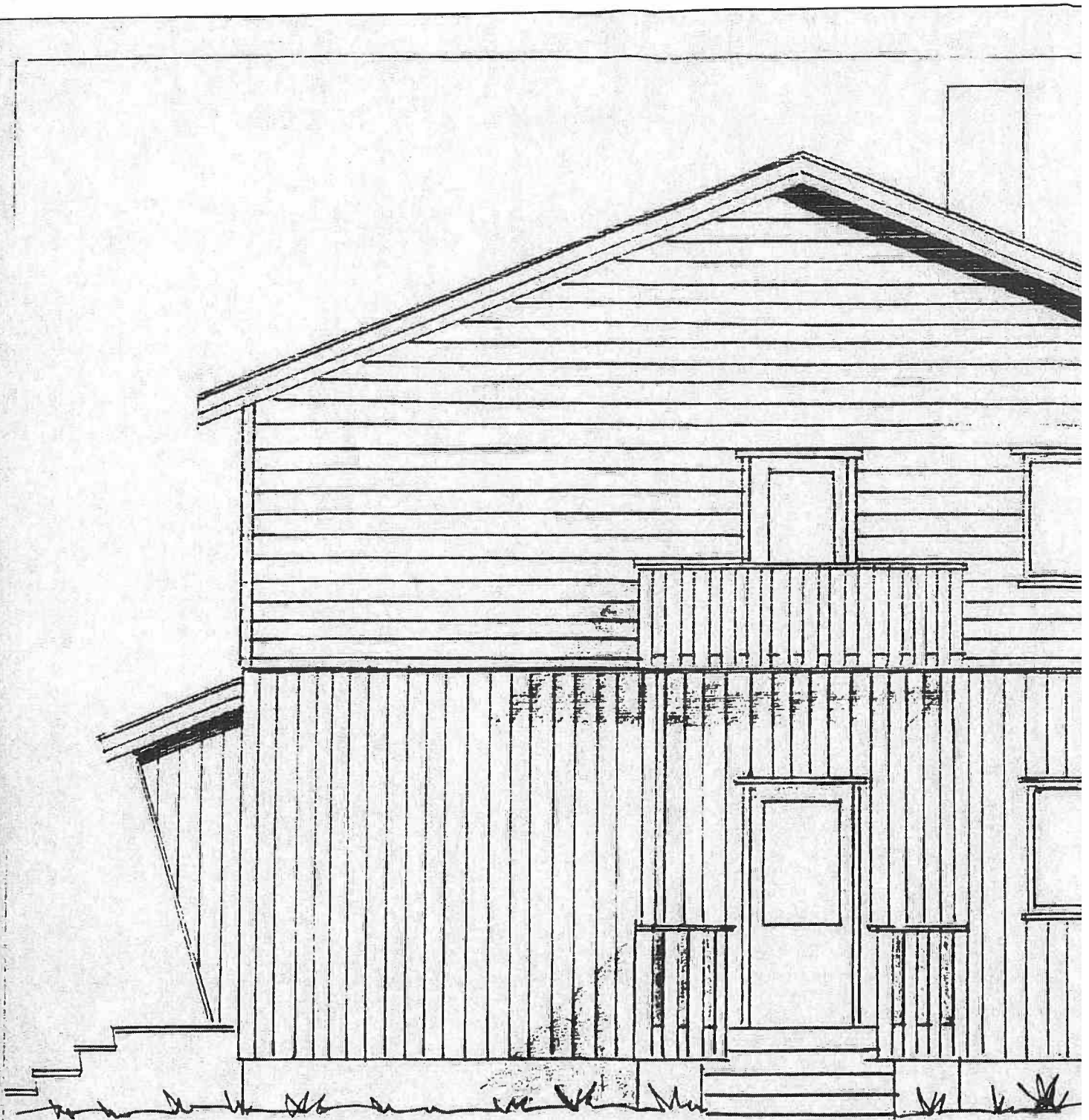
FASADE SYD
