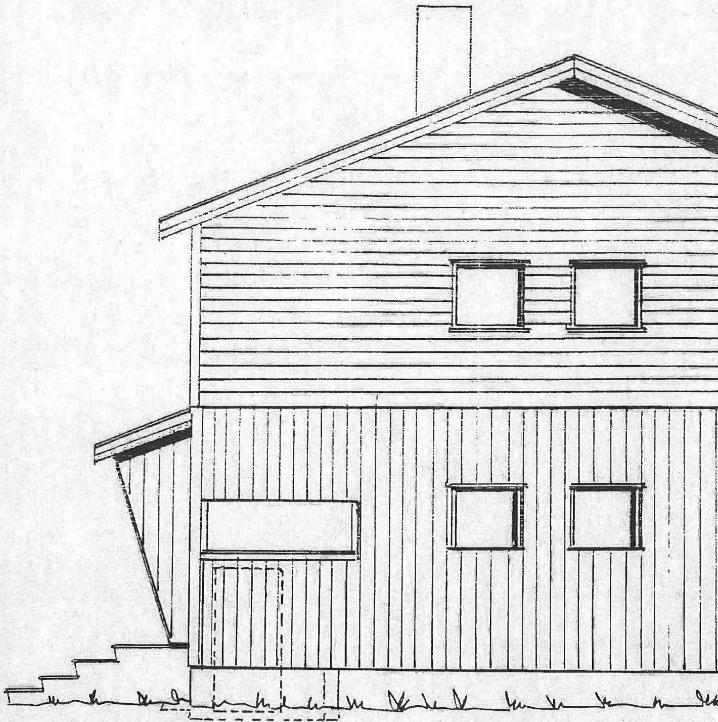
FASADE NORD
