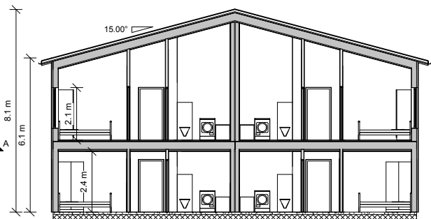
SNITT
