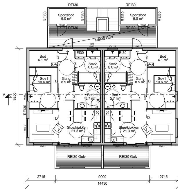
PLAN 2. ETASJE
