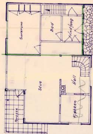
Plan 1 etg.
