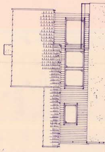
Vestvegg
