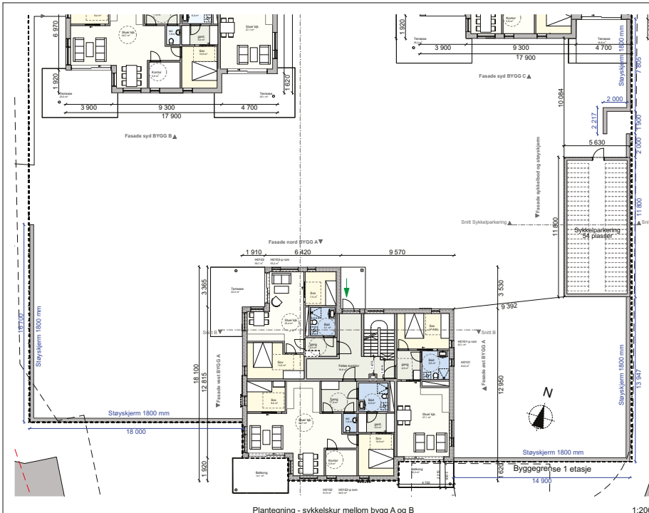
Plantegning - sykkelkur mellom bygg A og B 1:200
