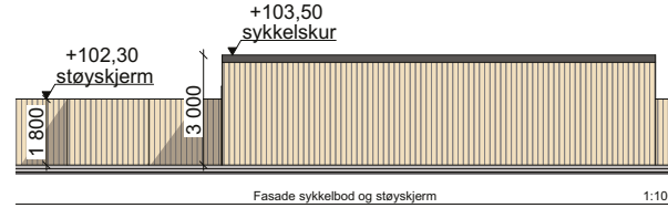
Fasade sykkelbod og støyskjerm 1:100
