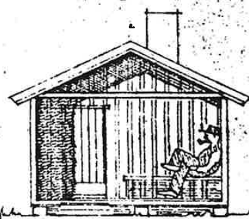
mot syd-øst GAVLFASADE HYTTE
