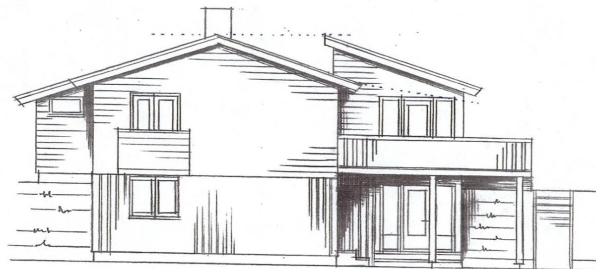
FASADE NORD
