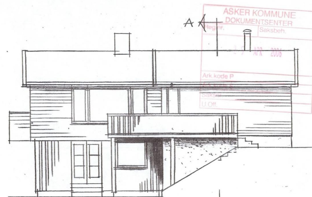
FASADE VEST
