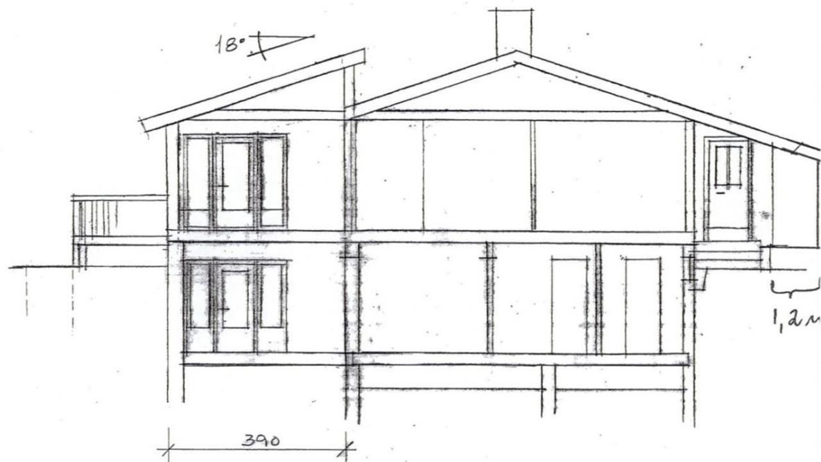
SNITT A-A
